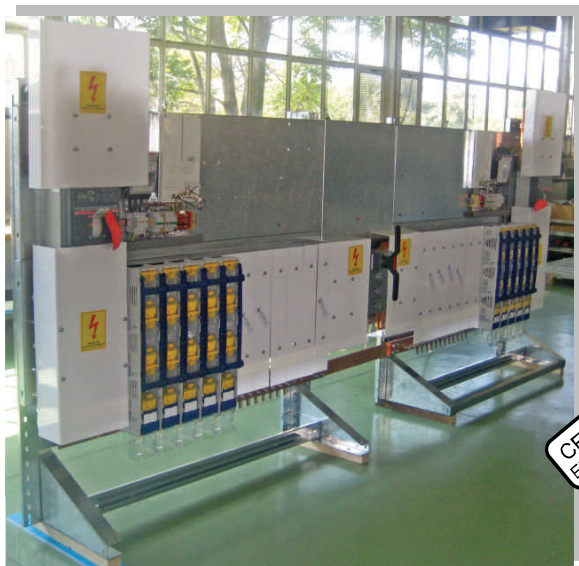
Нисконапонска табла 2x1000kVA со спојно поле 1600A
